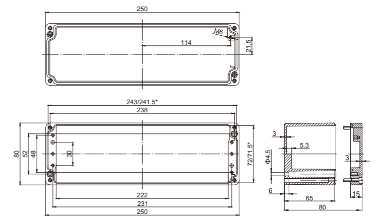
型號：DA172 重量：0.95kg 規格：80x250x80mm 卡軌型號和長度：TS15 -240mm
