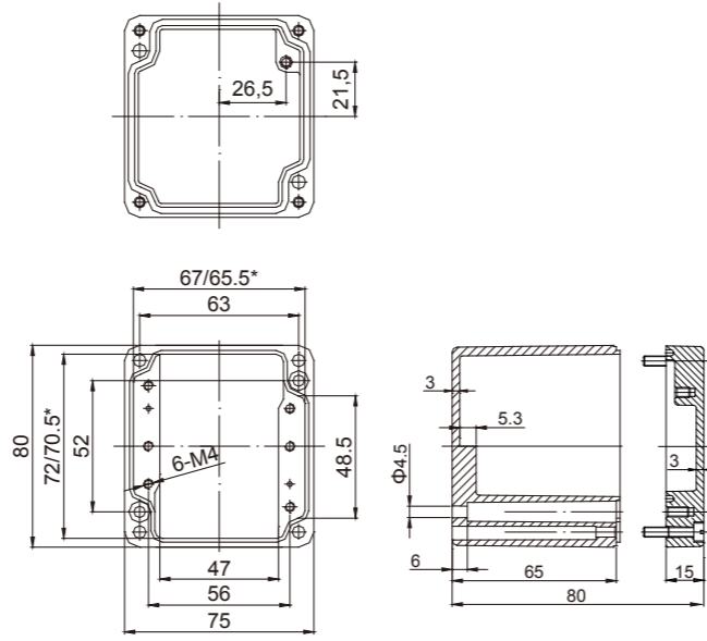
型號：DA142 重量：0.35kg 規格：80x75x80mm 卡軌型號和長度：TS15 -64mm
