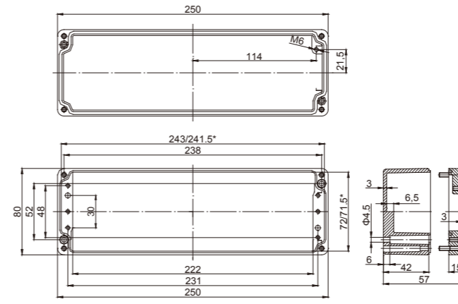
型號：DA171 重量：0.8kg 規格：80x250x57mm 卡軌型號和長度：TS15 -240mm
