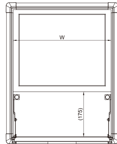
箱體寬度=顯示器寬度W+55 Body width= Display width+55
