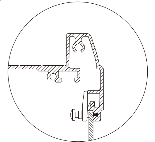
箱體左右側面板安裝
