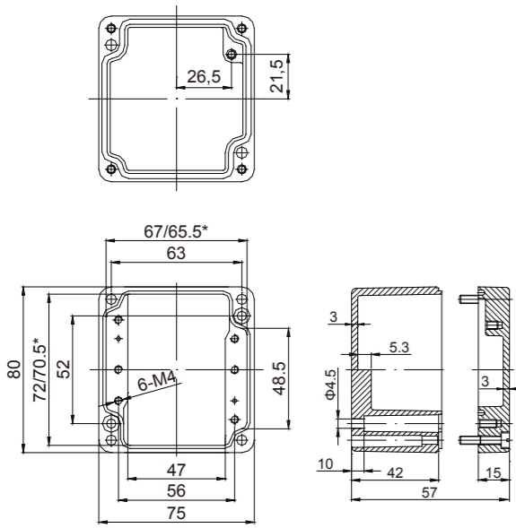
型號：DA141 重量：0.28kg 規格：80x75x57mm 卡軌型號和長度：TS15 -64mm
