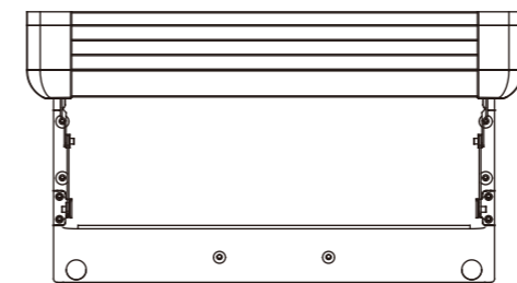
箱體寬度=顯示器寬度W+55 Body width= Display width+55
