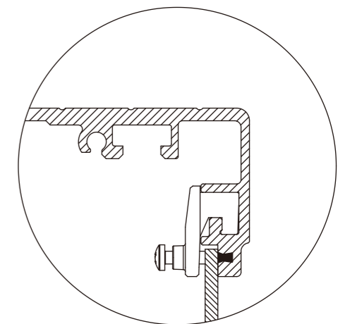
箱體上下側面板安裝
